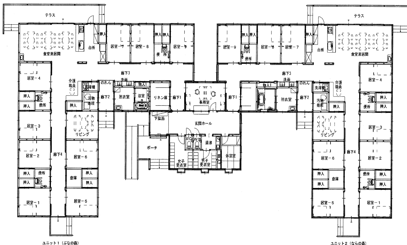
平面図
