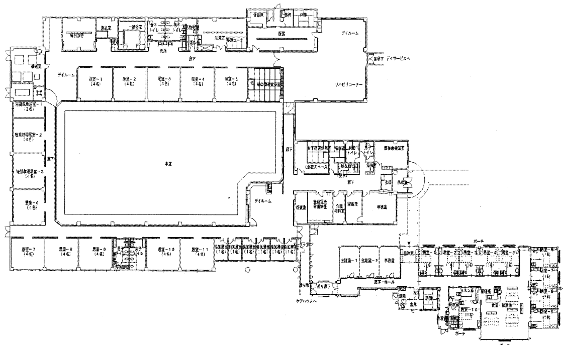
平面図
